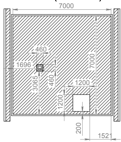
S-S (1 : 100)
