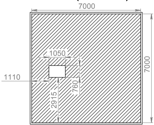
R-R (1 : 100)
