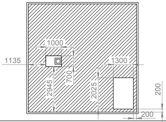
R-R (1 : 100)
